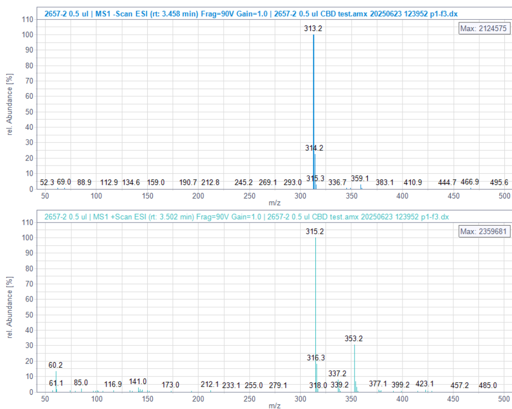
Рис. 7. Мас-спектри піку канабідіолу з часом утримування 3.5 хв на хроматограмі ацетонітрильного екстракту зразка № 2657/2 (-ESI зверху та +ESI знизу)
