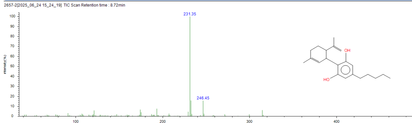
Рис. 10. Зареєстрована газова хроматограма ацетонітрильного екстракту зразка № 2657/2, зразка № 2657/1 та мас-спектр піку з часом утримування 8.7, котрий відповідає канабідіолу
