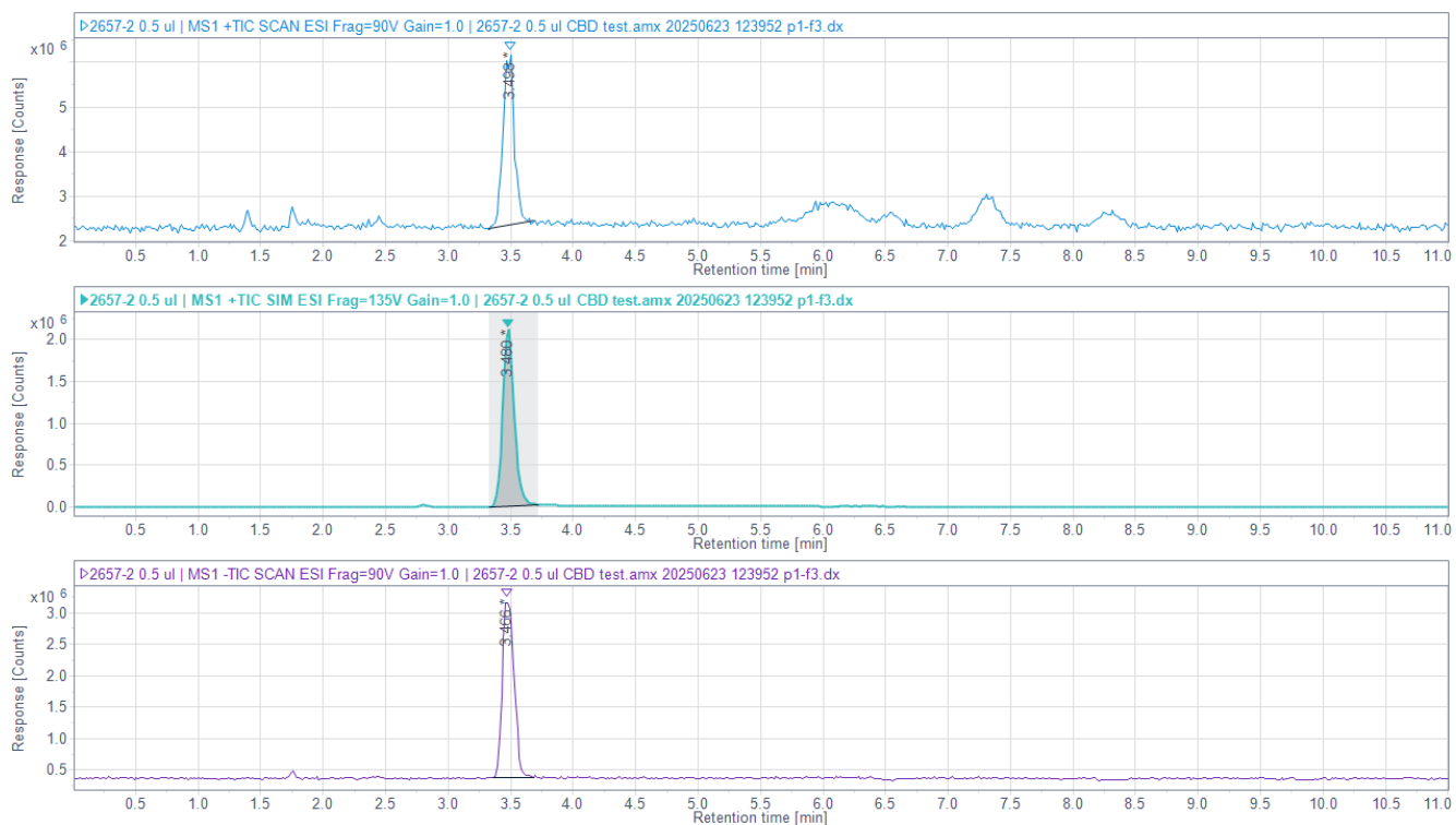
Рис. 4. Зареєстрована рідинна хроматограма ацетонітрильного екстракту зразка № 2657/2
