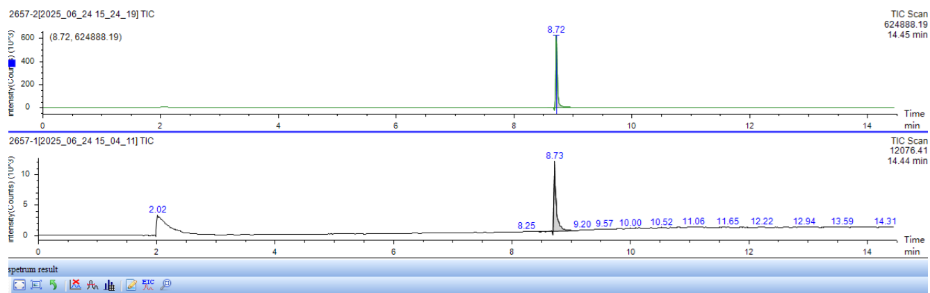
Рис. 9. Зареєстрована газова хроматограма ацетонітрильного екстракту зразка № 2657/2
